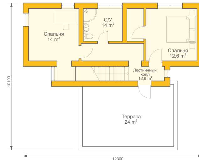
Экспликация | 2 этаж
