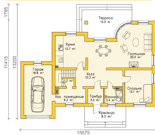
Экспликация | 1 этаж
