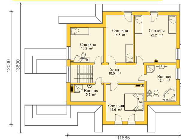
Экспликация | 2 этаж
